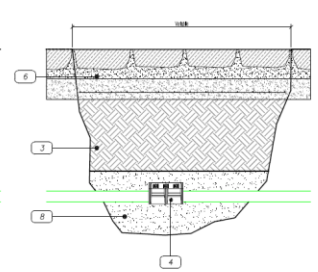
SEZIONE B-B
