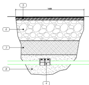
Sede stradale bitumata SEZIONE A-A
