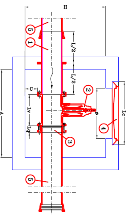
SEZIONE (1:20)
