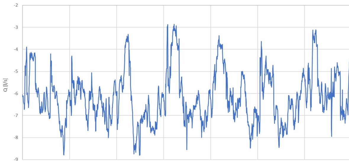
FIGURA 5-3: ESEMPIO DI GRAFICO CHE RAPPRESENTA L'ANDAMENTO DELLE PORTATE MISURATE IN CORRISPONDENZA DI UN PUNTO DI MISURA INSTALLATO IN RETE
